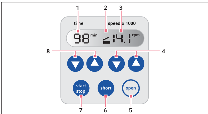
Рис. 5-1: Элементы управления MiniSpin/MiniSpin plus
