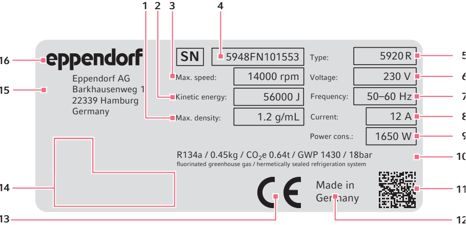
Рис. 3-1: Обозначение устройства Eppendorf AG (пример)
